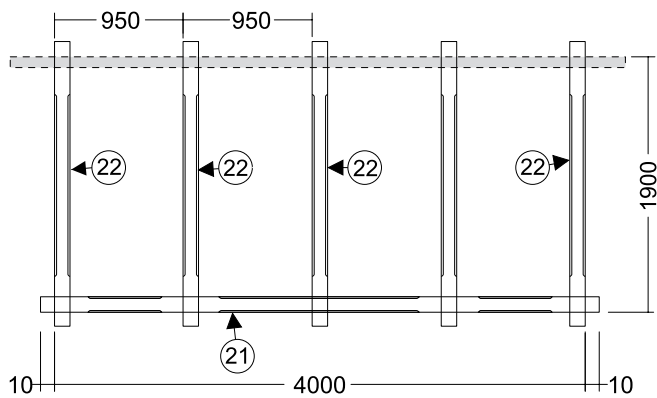
Bjelkelag sett undenfra
